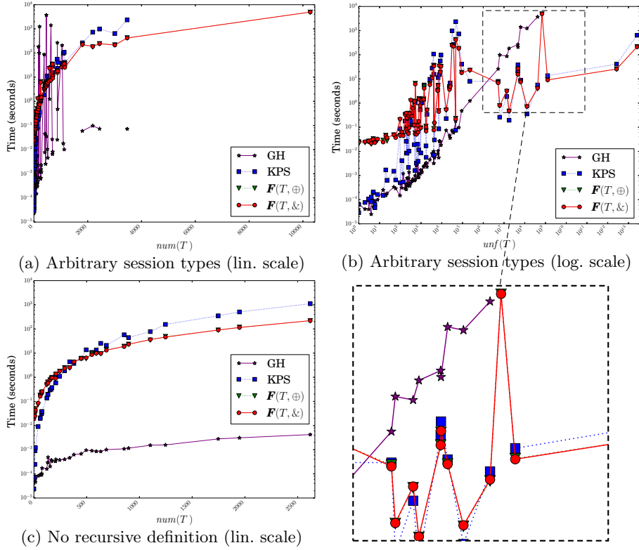
Fig. 3. Benchmarks (1)
